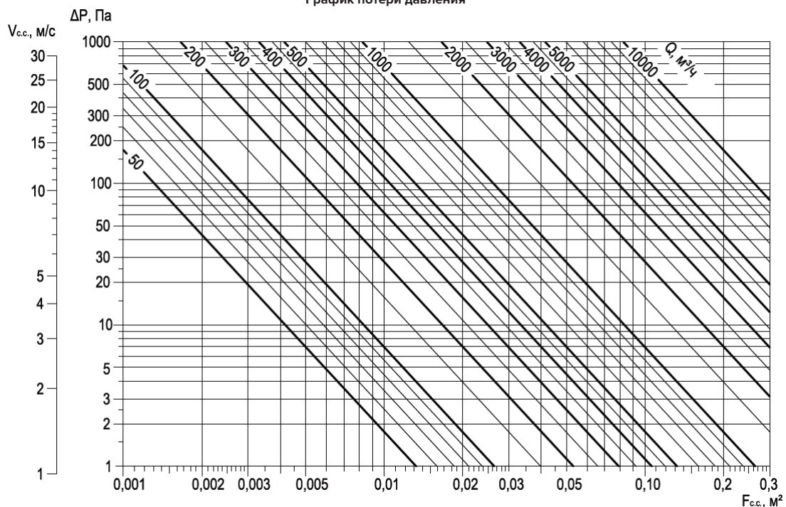
График потери давления
